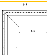
OC 61/90 Roh vnější 90°
