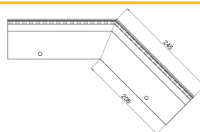
OC 61/135 Roh vnější 135°
