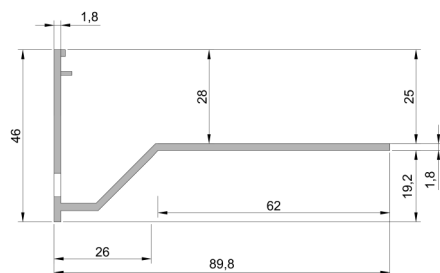
OC 61/90 Roh vnější 90°
