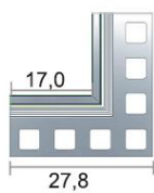
IC 61/90 Roh vnitřní 90°
